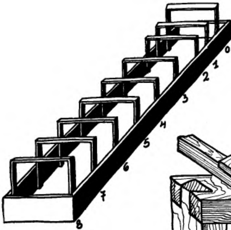
Abb. 114. Rumpfhelling.
