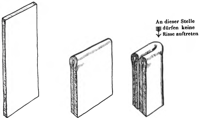
Abb. 8. Doppelte Faltprobe.
