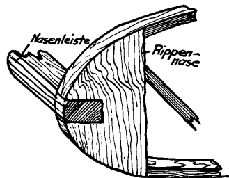
Abb. 92. Einbau der Nasenleiste Vorderkante der Leiste etwas mehr abrunden, als durch die Nasenform bedingt, damit sich die Leiste später nicht durch die Sperrholznase durchdrückt.
