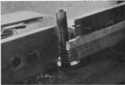
Abb. 39. Das Zuschneiden von Rippenleisten.
