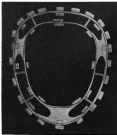
Abb. 69. Klotzschablone für runde Spante.
