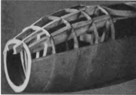
Abb. 129. Schablonenhölzer sind unter den Spanten eingepaßt.
