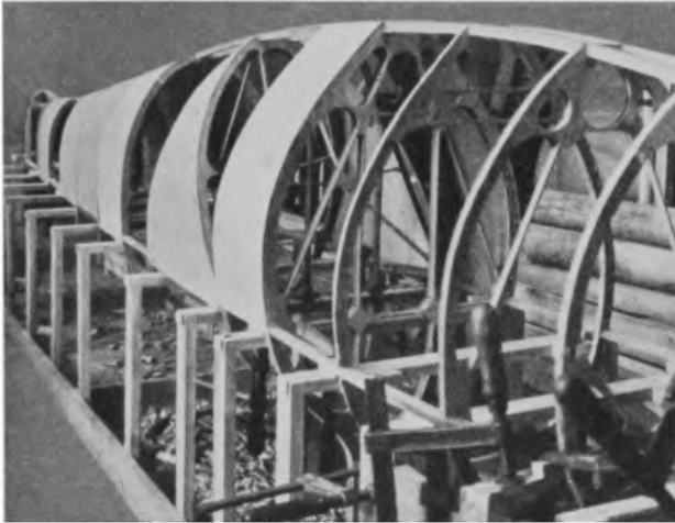
Abb. 112. Rumpfhelling.
