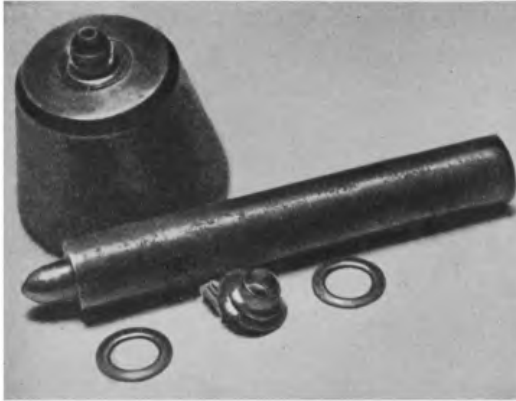
Abb. 4. Nietapparat.
