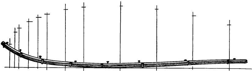
Abb. 40. Aufzeichnen der Rippenform mit Leiste und Nägeln.
