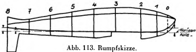
Abb. 113. Rumpfskizze.
