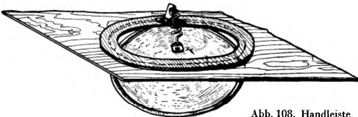
Abb. 108. Handleiste. Aluminiumdeckel mit Scharnier auf Flügeluntersatz befestigt. Die Feder hält die Klappen geschlossen. Am Rande des Deckels ist ein Draht zur Versteifung eingelegt.
