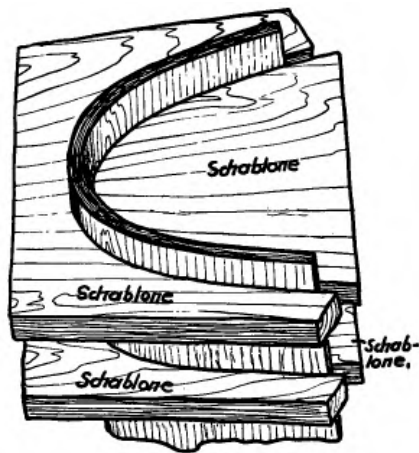
Abb. 72. Schablonen zum Verleimen der Nase.
