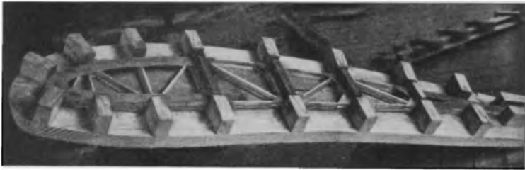
Abb. 48. Schablone für 2 – 3 Rippen.
