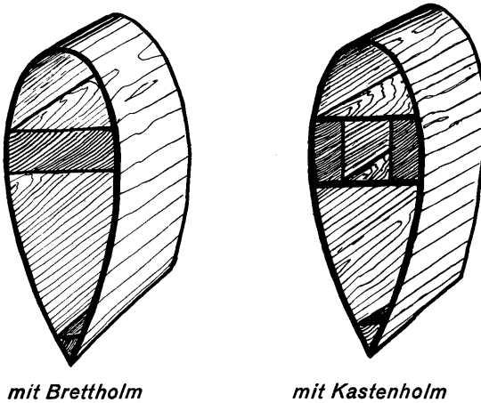
Abb. 142. Hohle Streben.
