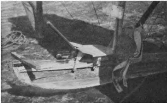
Abb. 123. Zöglingssitz.
