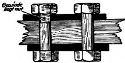
Abb. 81. Gewinde des linken Bolzen liegt tragend auf.
