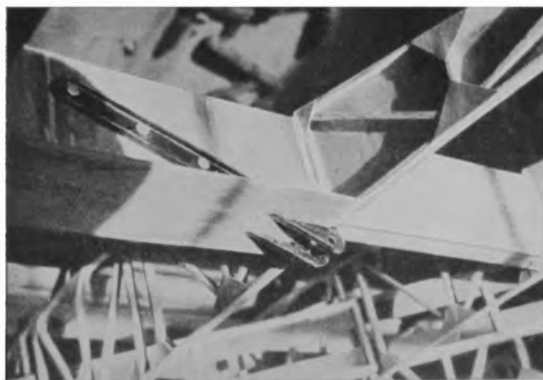
Abb. 105. Beschlagaustritt wird mit einer Sperrholzecke umgeben.
