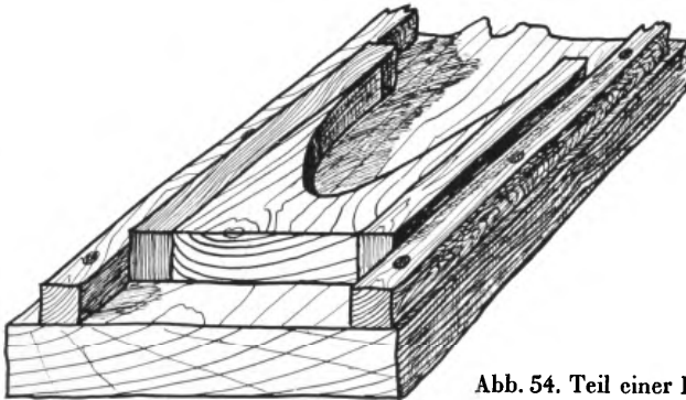
Abb. 54. Teil einer Holmschablone.
