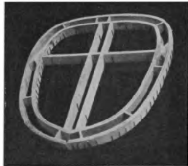
Abb. 68. Gebogenes Spant in einer Nagelschablone. Zu beachten sind noch die schwalbenschwanzförmig ausgeschnittenen Füllklötze.
