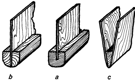
Abb. 66. Verschiedene Ausführungen von Randleisten.
