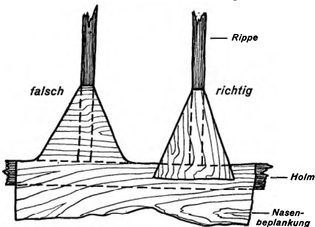
Abb. 104. Richtige und verkehrte Anbringung von Sperrholzecken.
