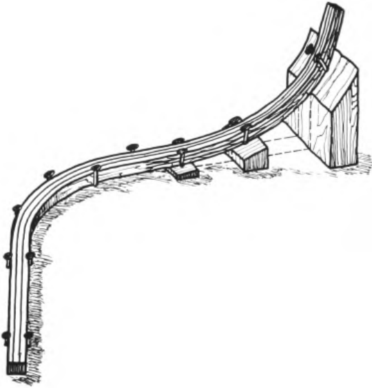
Abb. 64. Verleimen von räumlich gebogenen Leisten.
