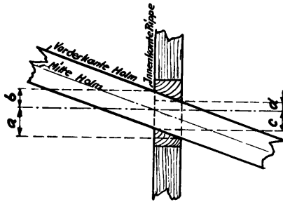
Abb. 91. Rippe und Holmkreuzung von oben gesehen.
