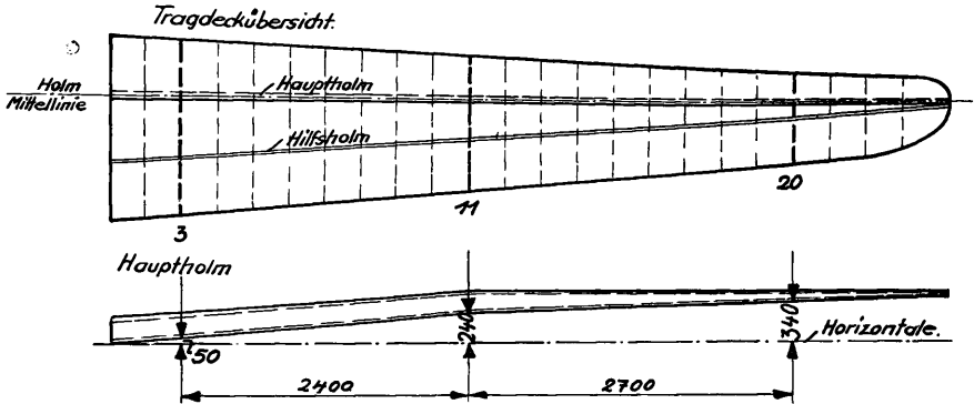
Abb. 84. Tragdeckübersicht mit Holzzeichnung. Der Holm ist bei Rippe 11 geknickt.
