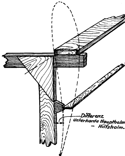
Abb. 89. Schematische Darstellung von Rippe und Holm auf der senkrechten Stellung.
