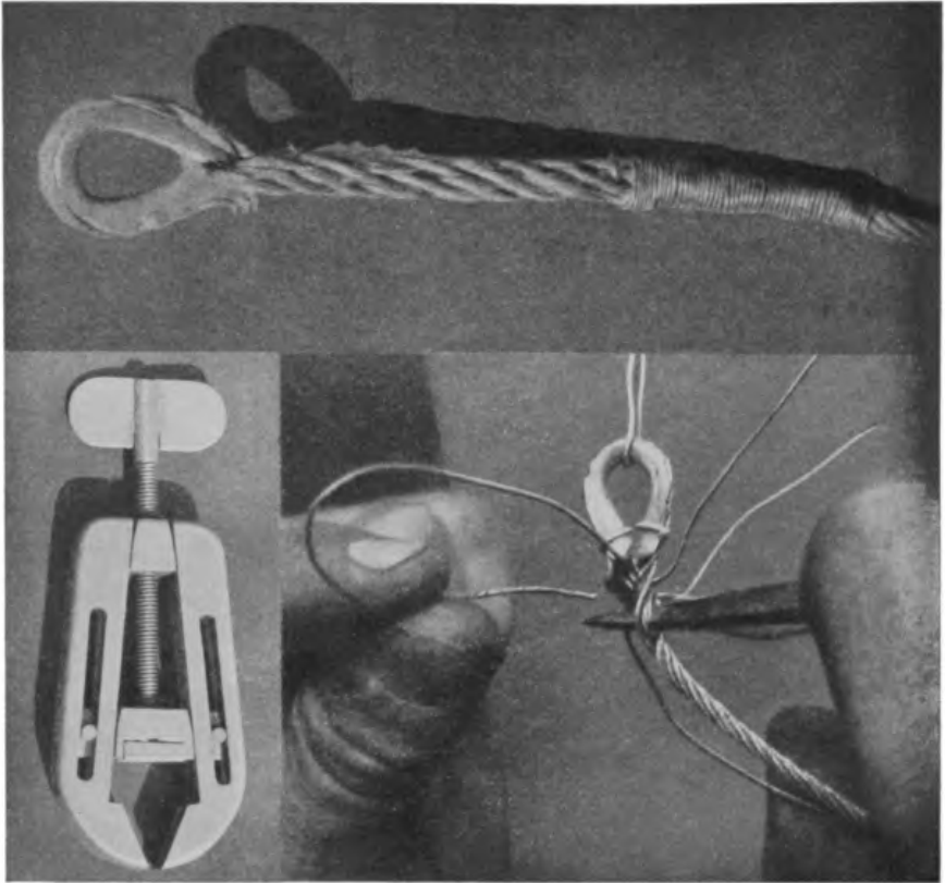
Abb. 25. Spleißkluppe.
