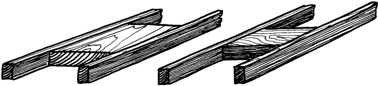
Abb. 57. Füllklötze, wie sie nicht eingebaut werden sollen, da sie keinen weichen Übergang vom Klotz in den Gurt haben.
