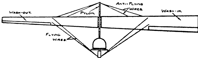
FIG. 14.—Truing up Glider.
