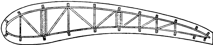
FIG. 33.—Rib Jig.
