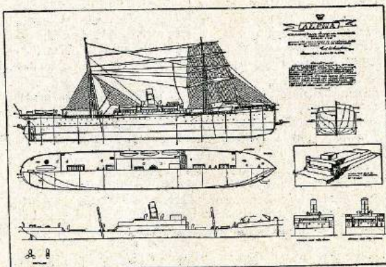
SF. 5. Ångfartyget "Alpha".
