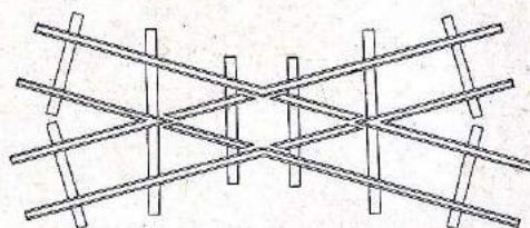
FÄRDIGBYGGDA VÄXLAR (Hö). HÖGER OCH VÄNSTER.
