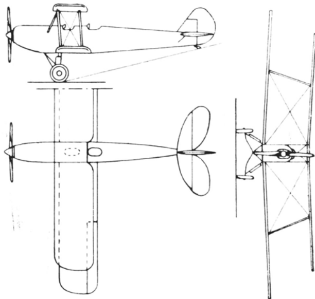
Caproni CA 100
