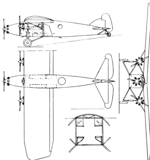
Caproni CA 101 - Trasporto truppe e feriti.
