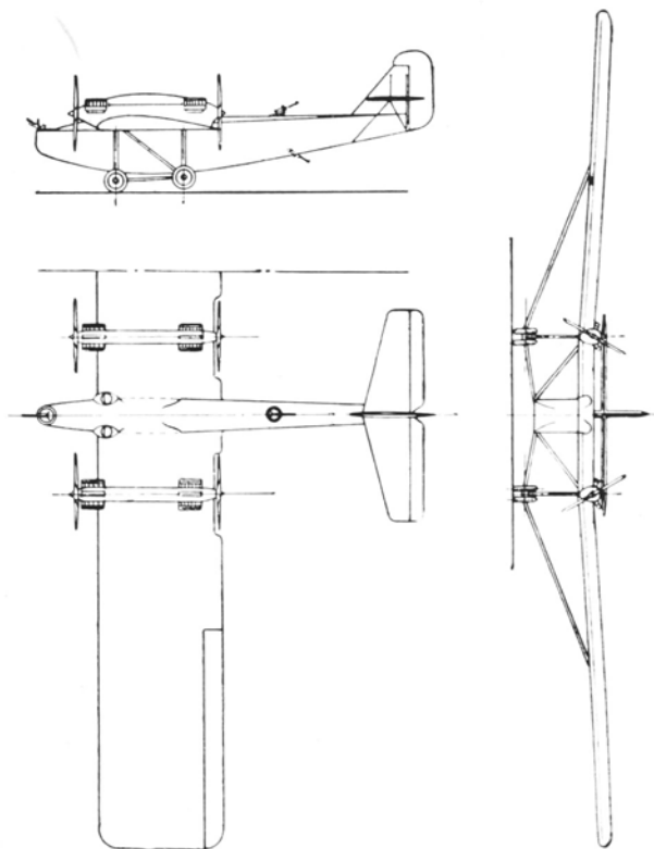
Caproni CA 94
