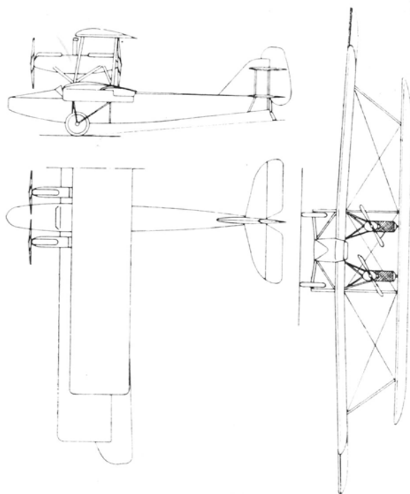
Caproni CA 87
