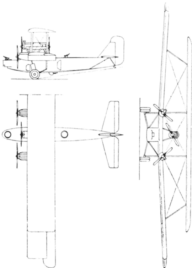
Caproni CA 79
