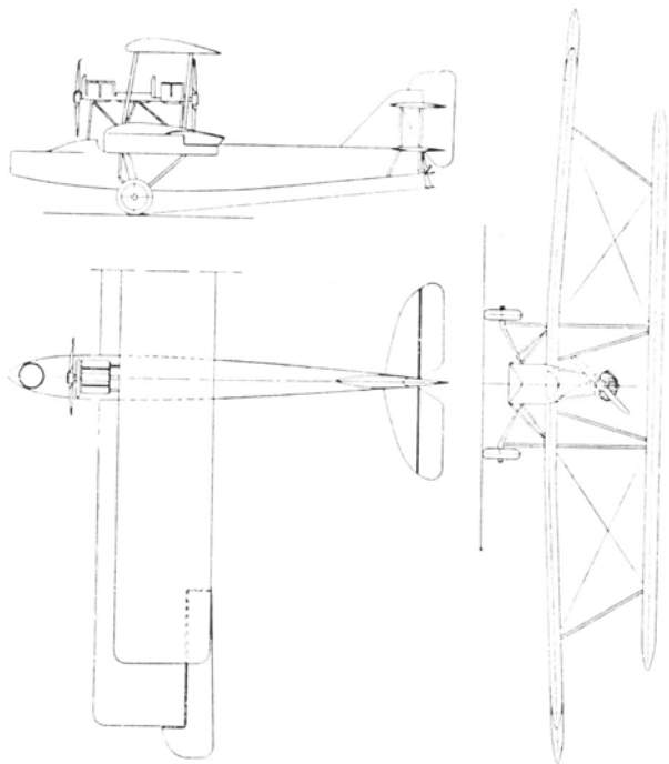
Caproni CA 78
