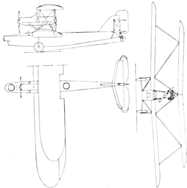
Caproni CA 103
