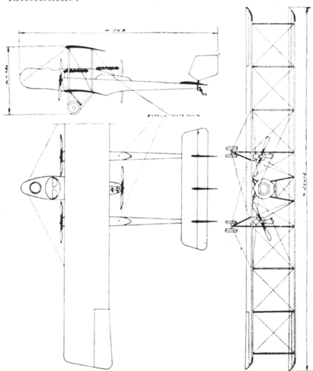
Caproni CA 50
