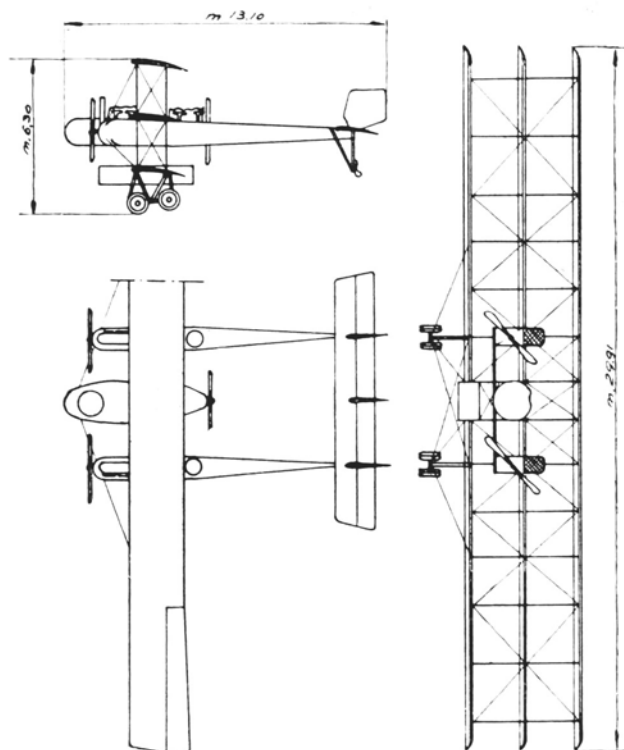
Caproni CA 42
