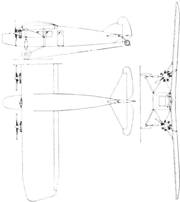
Caproni CA 102
