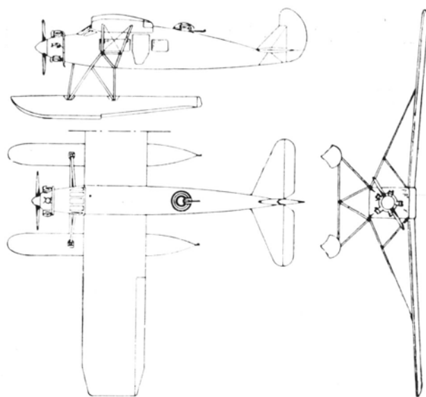
Caproni CA 97 idro.
