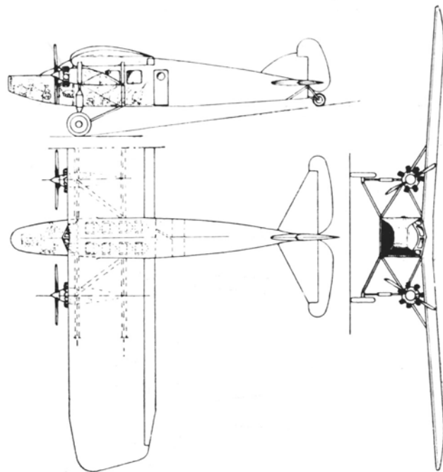
Caproni CA 102 Civile
