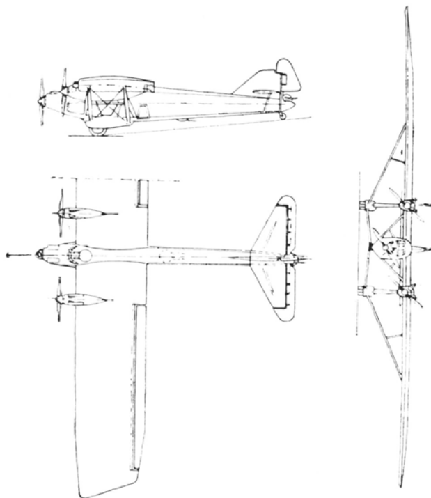
Caproni CA 95
