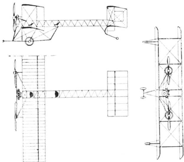
Caproni CA 1
