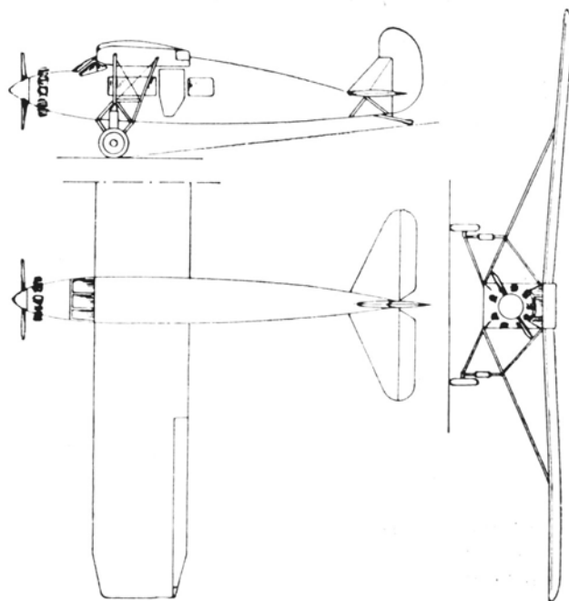
Caproni CA 97 monomotore
