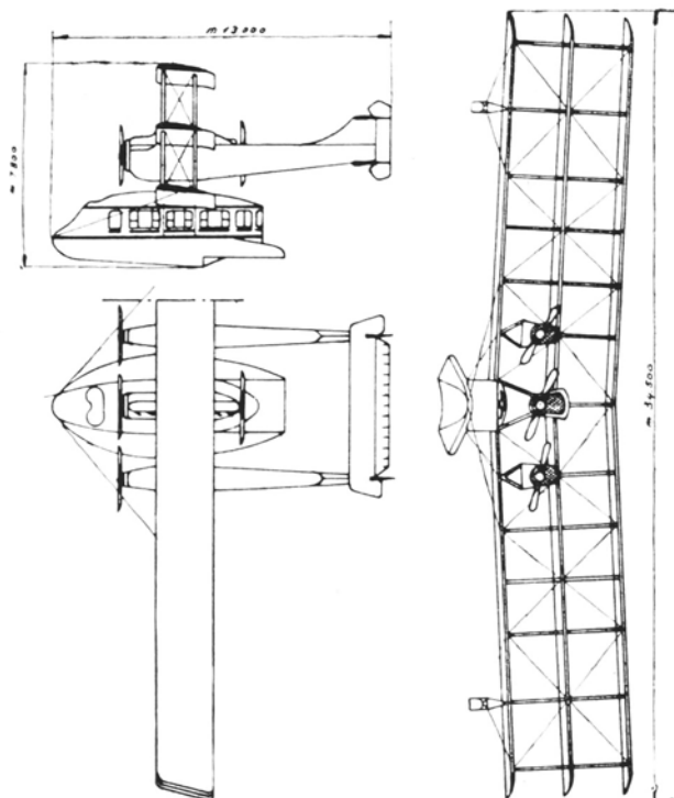
Caproni CA 49
