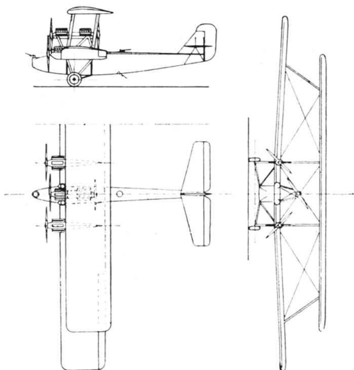
Caproni CA 96
