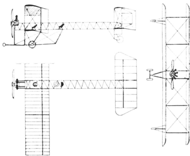
Caproni CA 2
