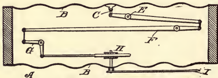
Fig. 74. Aneroid Barometer.
