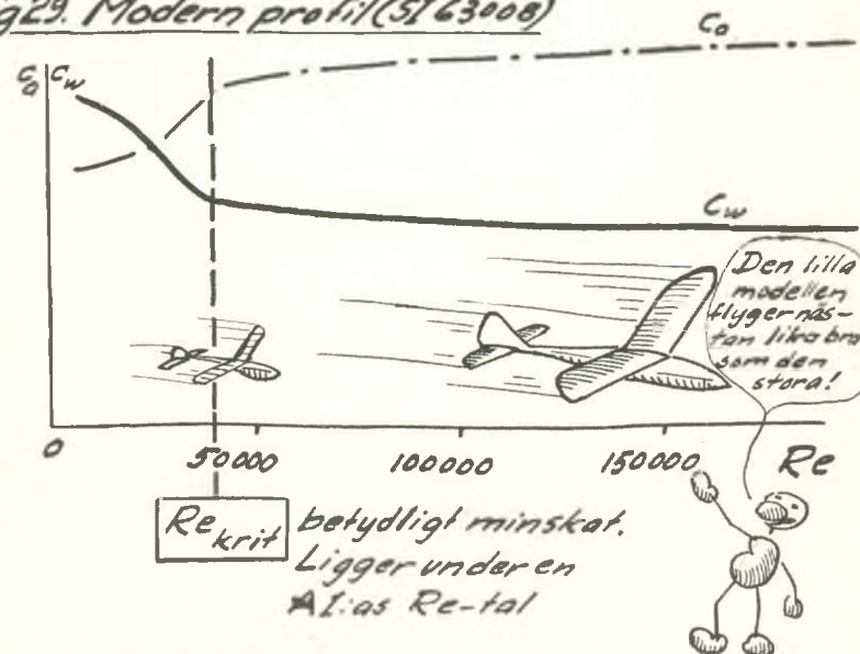
Fig. 29. Modern profil (SI 63008)
