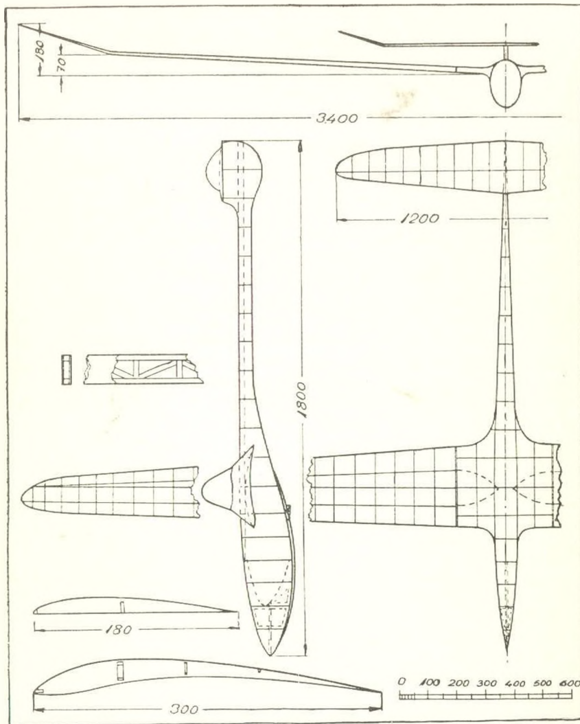
Detta är kanske den förnämsta segelmodell som byggts i världen, den finska "Kuha 15" med spv. 340 cm, en vingyta av 71 dm 2 och en vingbelastning av 22 g/dm 2 . Genom sin storlek har modellen ett högt reynoldstal trots sitt excellenta sidoförhållande av 1:17, vilket annars vore omöjligt att använda. "Kuha 15" uppges också ha ett glidtal av 28, vilket är dubbelt så högt som det bästa uppnådda hos "normala" modeller. Sjunkhastigheten torde ligga mellan 0,20 och 0,25 m/sck! Med sin effektiva V-form och sin ytterst ringa fenyta är modellen en självupprätande typ.
