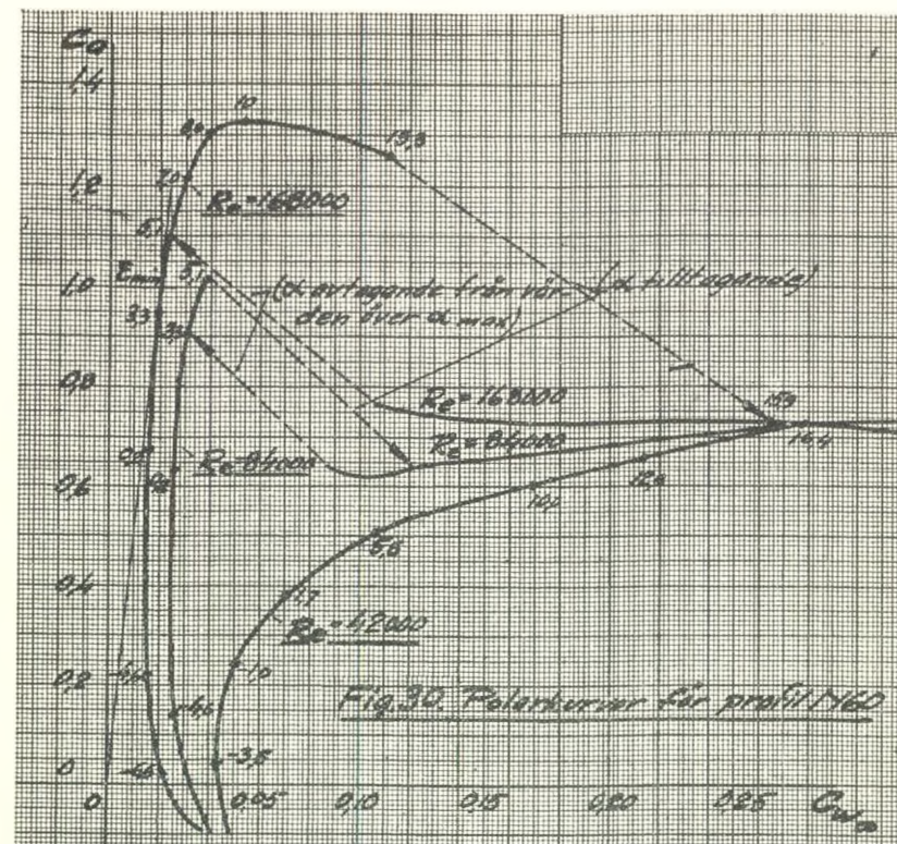
Diagrammet visar polarkurvor för N 60 vid olika Re -tal. Nedåtriktad, streckad pil anger övergång från över- till underkritisk strömning vid ökande \alpha . Uppåtriktad pil visar hur strömningen blir överkritisk vid avtagande anfallsvinkel. Märkligt nog håller sig som synes strömningen underkritisk längre ned på \alpha -skalan, då \alpha minskas.
