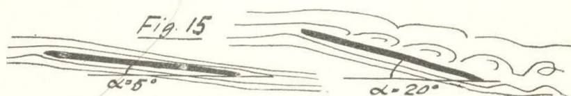
Vänstra bilden visar hur luftströmmen följer plattan vid \alpha = 5^\circ . T. h. har \alpha_{max} uppnåtts. Strömmen avlöses och bildar virvlar åstadkommande ett stort motstånd.
