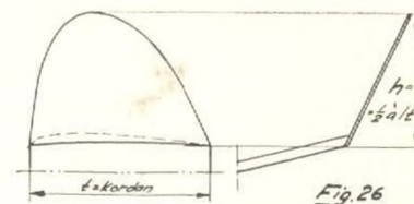
Fig. 26 Vingöra. Effektiviteten med avseende på spetsutjämnningen ökar med örats höjd, men då höjs också lateralcentrum.
