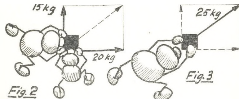
Pojkarna trycker på lädan med 15 och 20 kg krafter, vinkelrätt mot varandra. Lädan åker då iväg i diagonalens riktning.
