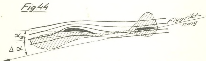
Plane! intar därför detta läge i glidflykten, d. v. s. kropp och vinge får \Delta\alpha^\circ högre anfallsvinkel ( \Delta\alpha = nedsvepningsvinkeln).
