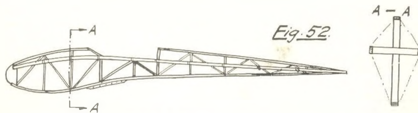
Fig. 52. Korsspantkropp med diagonalförstärkning i det platt byggda, vertikala formskelettet. På detta limmas horisontella tvärlister (spant), mot vilkas ändar sidolongerongerna limmas (se sektionen t. h.!).
