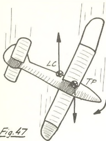
Då LC ligger långt bak blir modellen också ostabil genom att gå ur kurs vid sidokaning.
