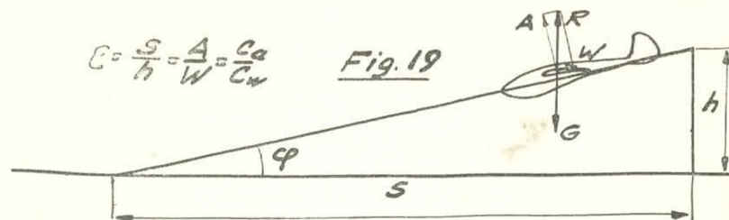
Fig. 19. Ett flygplan glider sträckan s från höjden h . Genom triangelarnas likformighet blir förhållandet detsamma (lyftkraft/motståndet).
