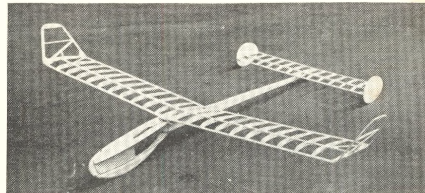
KSAK-3 "Sunnanvind" är beräknad som självupprätande modell. Obs. den stora framkroppen, de små fenorna och den kraftigt tvärstabiliserande V-formen med öron! Modellen illustrerar stävigheten att på ritningen beräkna fenytan rätt, i det den efter provflygning måste förses med 30 % större fena för att inte pendla i starten. "Sunnanvind" har med sin höga kurs- och tvärstabilitet visat sig vara en charmant hangmodell.
