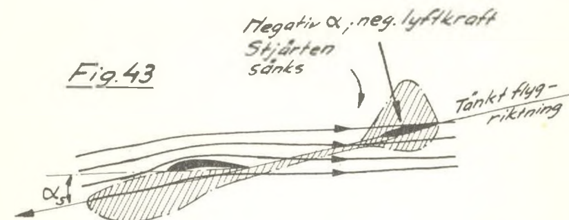
Om flygplanet skulle flyga i stabilisatorns 0 riktning, skulle nedsvepningen bakom vingen sänka stjärten.
