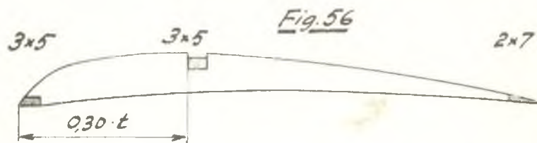
Profil: 63008, t=140 mm, Sprygel av 08 mm asp.
