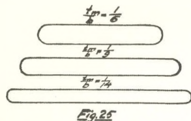
Fig. 25 Sidoförhållanden. 1/6 är det sämsta användbara för Y = 15 \text{ dm}^2 och 1/14 det "bästa" användbara för stora modeller ( Y = 70 \text{ dm}^2 ).
