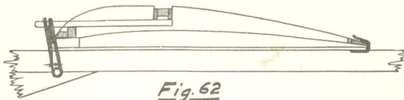
Enkel och effektiv ringfästning. Bakkanten hålls i läge av en bygge av t. x. en hårnål. Främre delen kan byggas in för att minska motståndet.
