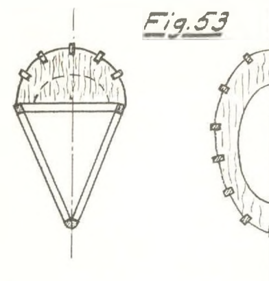
Fig. 53. Runda kroppssektioner. T. v. trekantig kropp med övre påbyggnad av halvcirkel-spant och formlistor. T. h. oval spantkropp i två halvor, vilka efter byggandet limmas ihop. Bägge kroppstyperna kan "plankas" med balsafanér.
