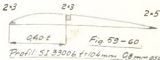
Ungefärliga dimensioner för segelmodellstyrverk.
