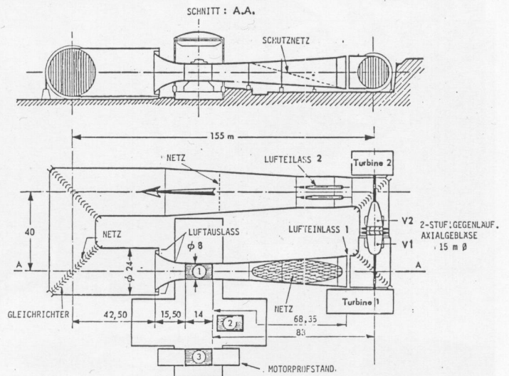
BILD 1: GESAMTSICHT DES GROSSEN HOCHGESCHWINDIGKEITS - WINDKANALS VON ÖTZTAL
