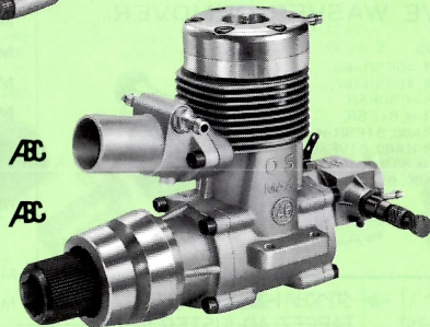
MAX-20FP-M (フライホイールは別売) (Flywheel is optional extra.)
