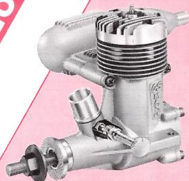
MAX-40FP-S MAX-35FP-S
