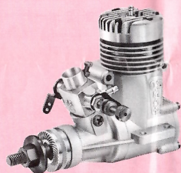
MAX-28F
