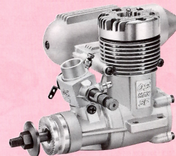
MAX-46SFÆ MAX-46SF
