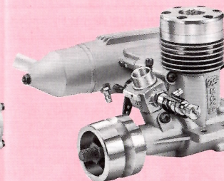
MAX-20FP-M (フライホイールは別売) (Flywheel is optional extra.)
