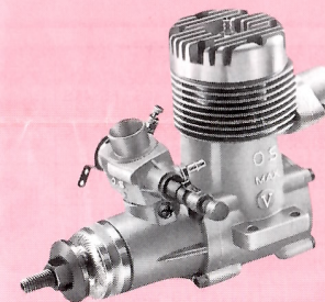
MAX-40VF Æ
