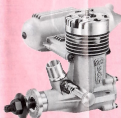
MAX-25FP-S MAX-20FP-S
