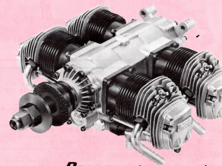
Pegasus (FF-240)
