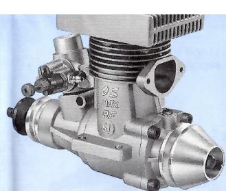
MAX-61RF-HS Æ MAX-61RF-HS
