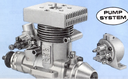
MAX-61RF-H Æ-P MAX-61RF-H-P
