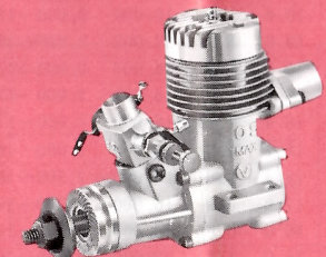
DUCTED FAN MAX-25VF-DFÆ MAX-25VFÆ
