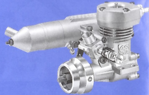
MAX-10FP-M (フライホイールは別売) (Flywheel is optional extra)
