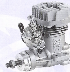
MAX-CZ-R エアクリナー付 (Supplied with Air Cleaner)
