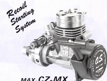
MAX-CZ-MX (フライホイールは別売) (Flywheel is optional extra)
