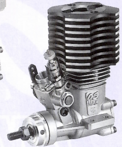
MAX-CZ-12Z エアクリナー付 (Supplied with Air Cleaner)
