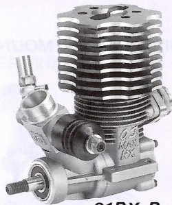
MAX-21RX-B エアクリナー付 (Supplied with Air Cleaner)
